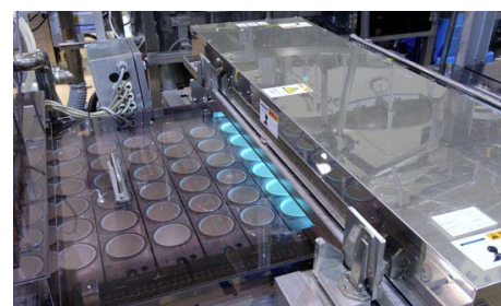
充填前の容器の表面殺菌 高出力表面殺菌装置400W×6灯用
