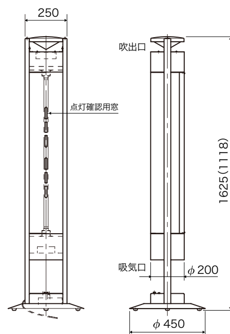
エアーリア30Wタイプ ※( )内は15Wタイプの寸法です。
