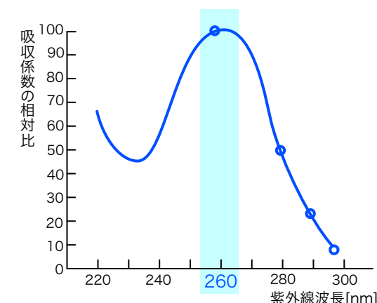
■ 細菌のDNAの分光特性
